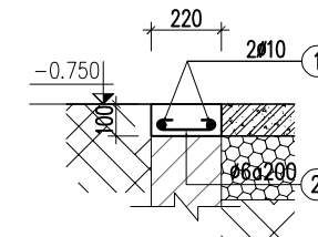
GT.2
