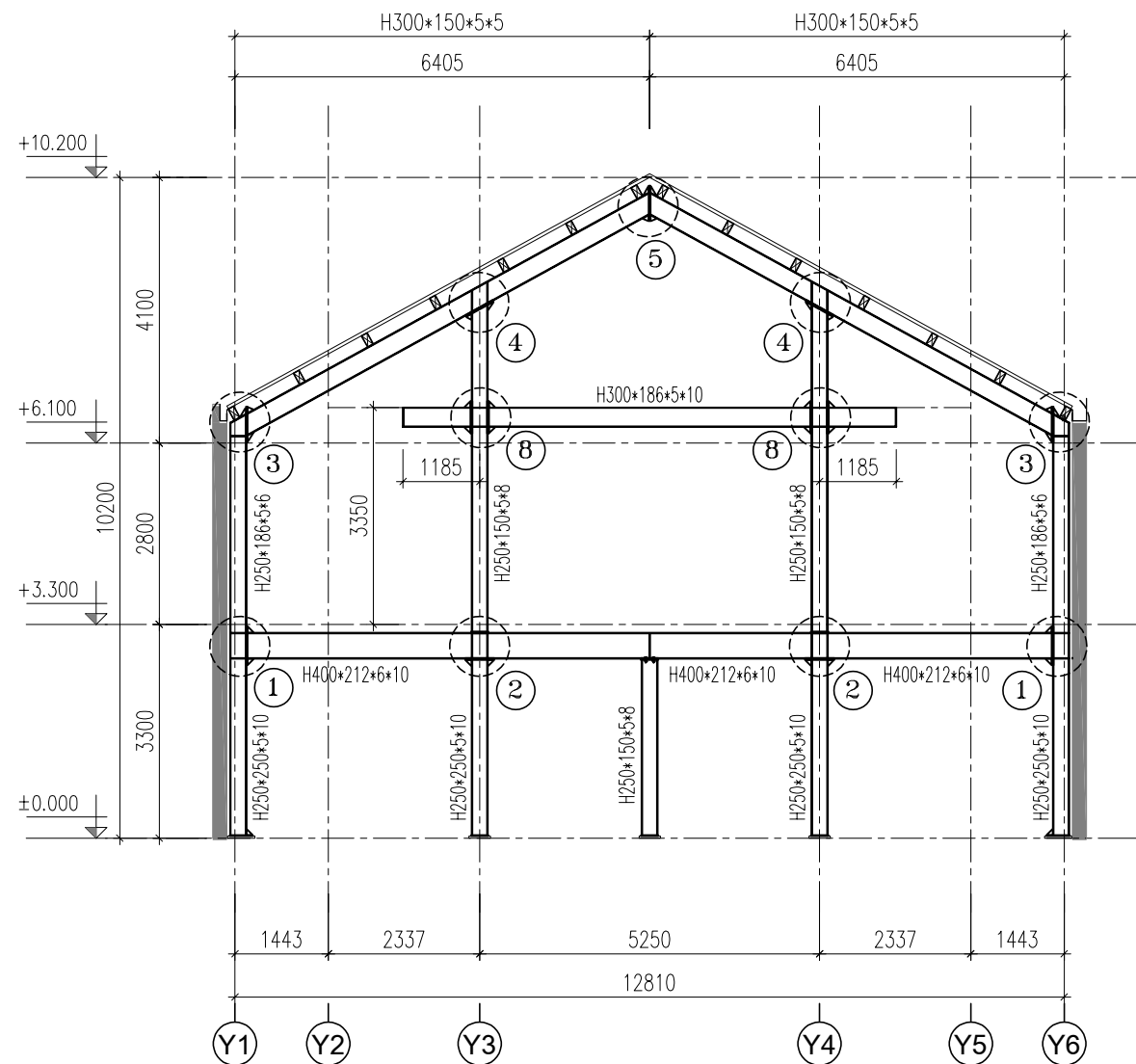
MẶT CẮT KHUNG MF1A
