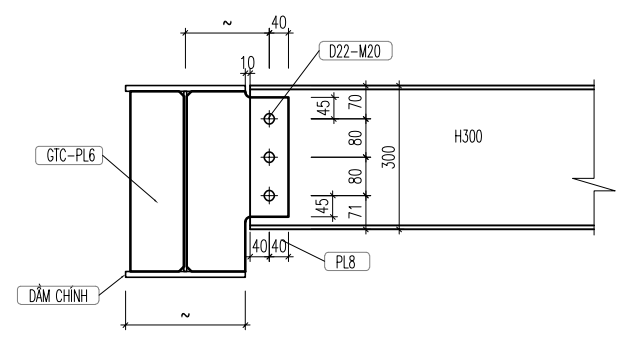
CHI TIẾT LIÊN KẾT DẦM PHỤ CHIỀU CAO H=250
