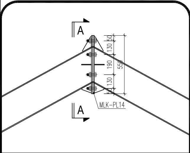
CHI TIẾT 5
