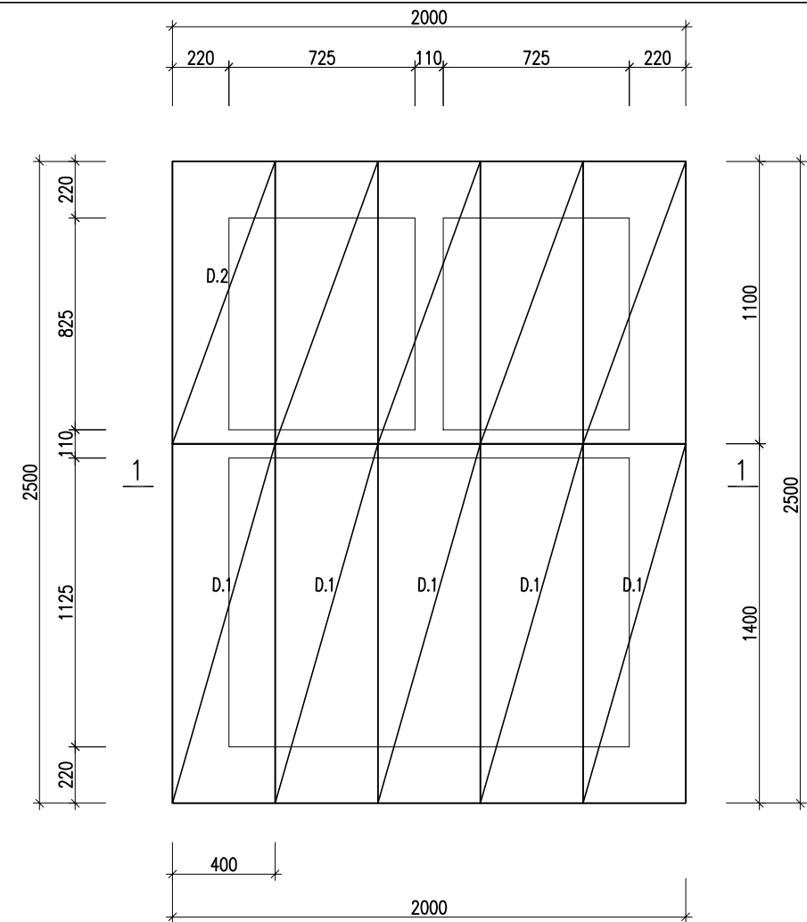
MẶT BẰNG BỐ TRÍ TẦM ĐÀN NẮP BỀ PHỐT
