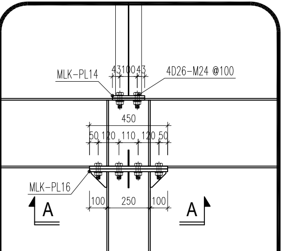
CHI TIẾT 6
