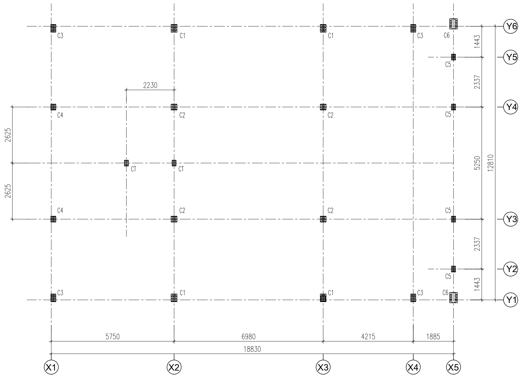
MẶT BẰNG CHÂN CỘT THÉP
