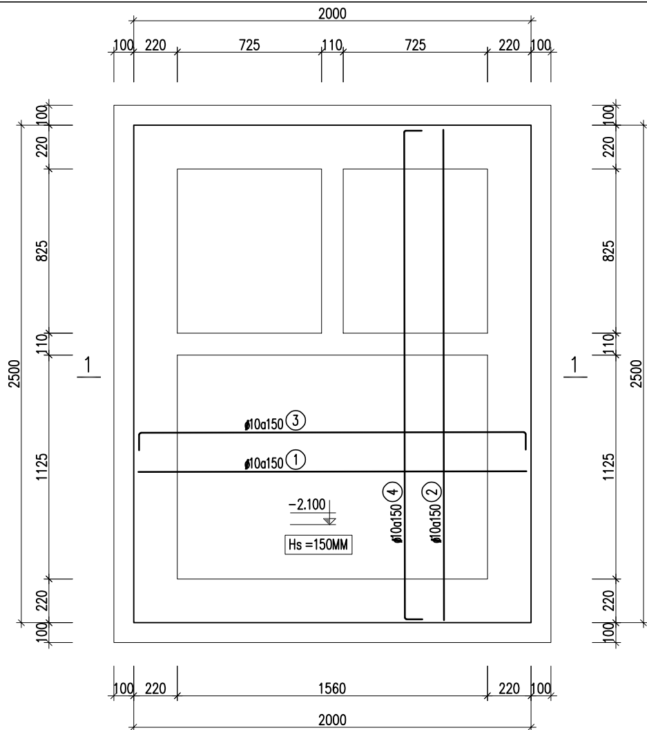
MẶT BẰNG BỐ TRÍ THÉP ĐÁY BỀ PHỐT
