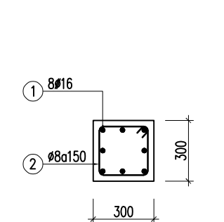
CM.1
