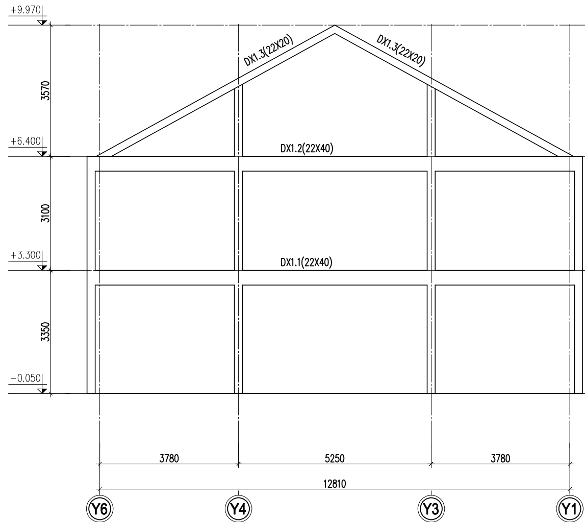
MẶT ĐỪNG KHUNG TRỤC X1
