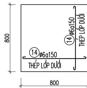
CHI TIẾT NẮP LỖ THĂM
