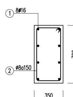
CM.7
