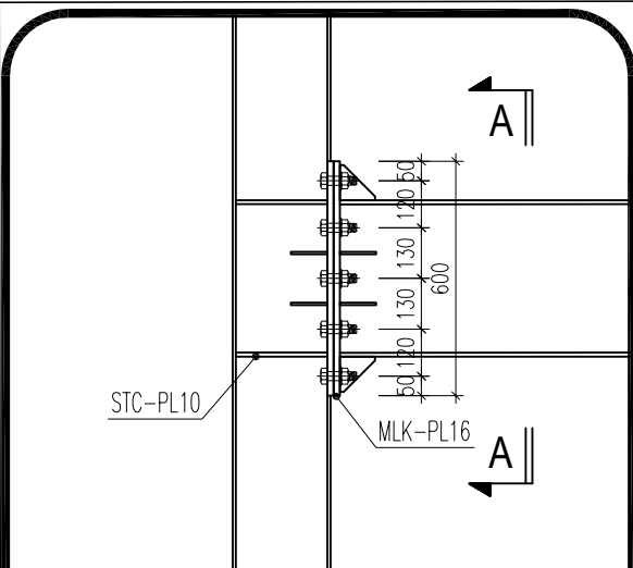
CHI TIẾT 1
