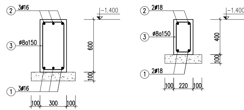
GM.1
