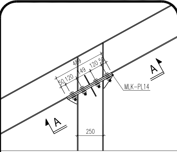
CHI TIẾT 4
