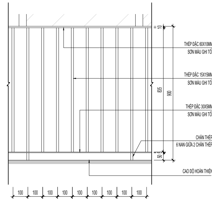
CHI TIẾT LAN CAN
