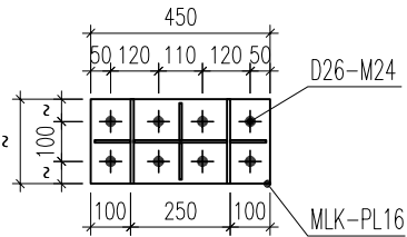
MẶT CẮT A-A
