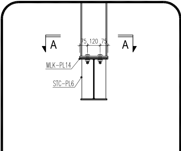
CHI TIẾT 10
