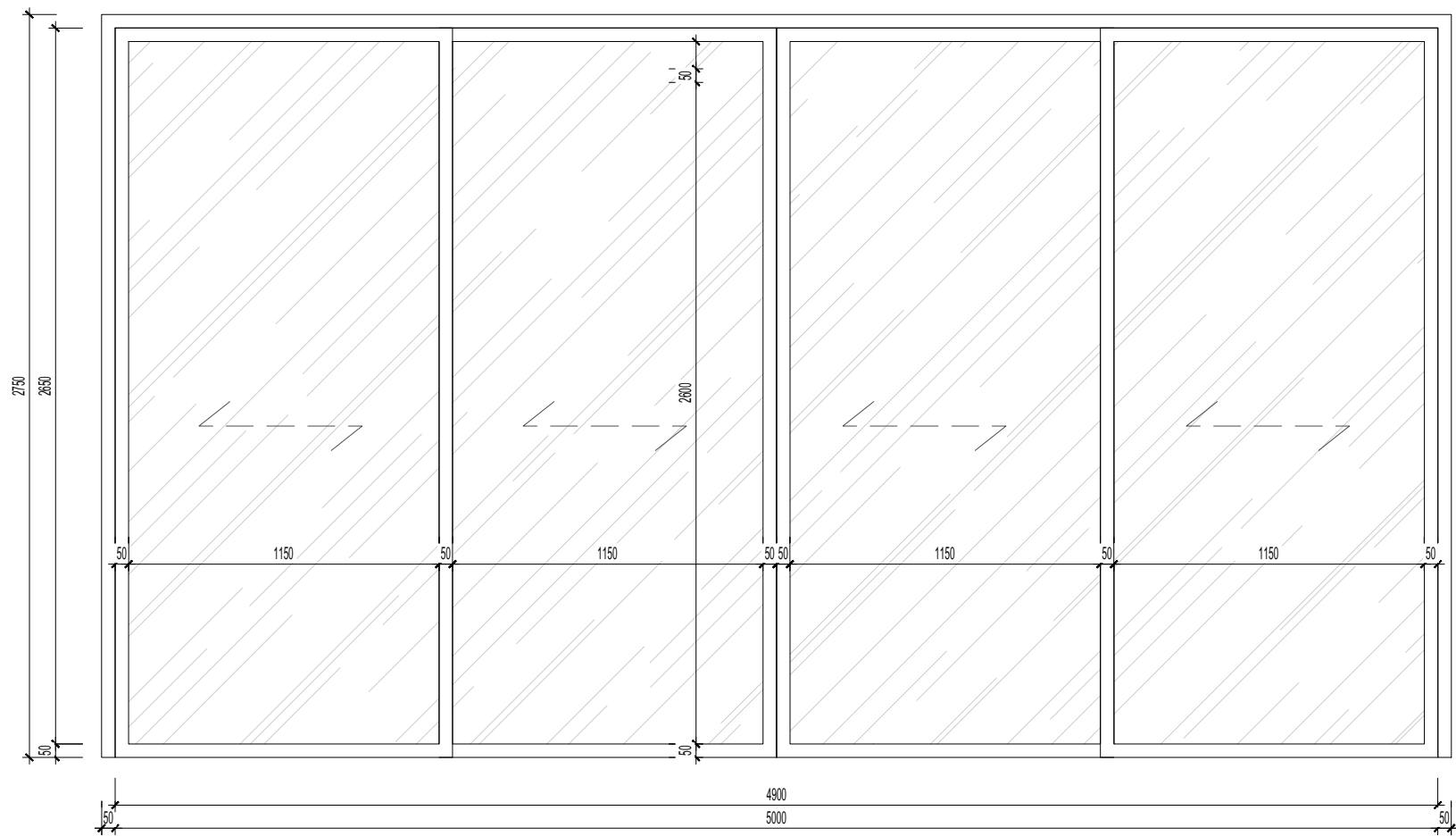
D1 - 5000X2750 - CỬA NHÔM KÍNH MỞ TRƯỢT - SL 1
