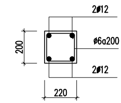
GIẺNG TƯỜNG 220
