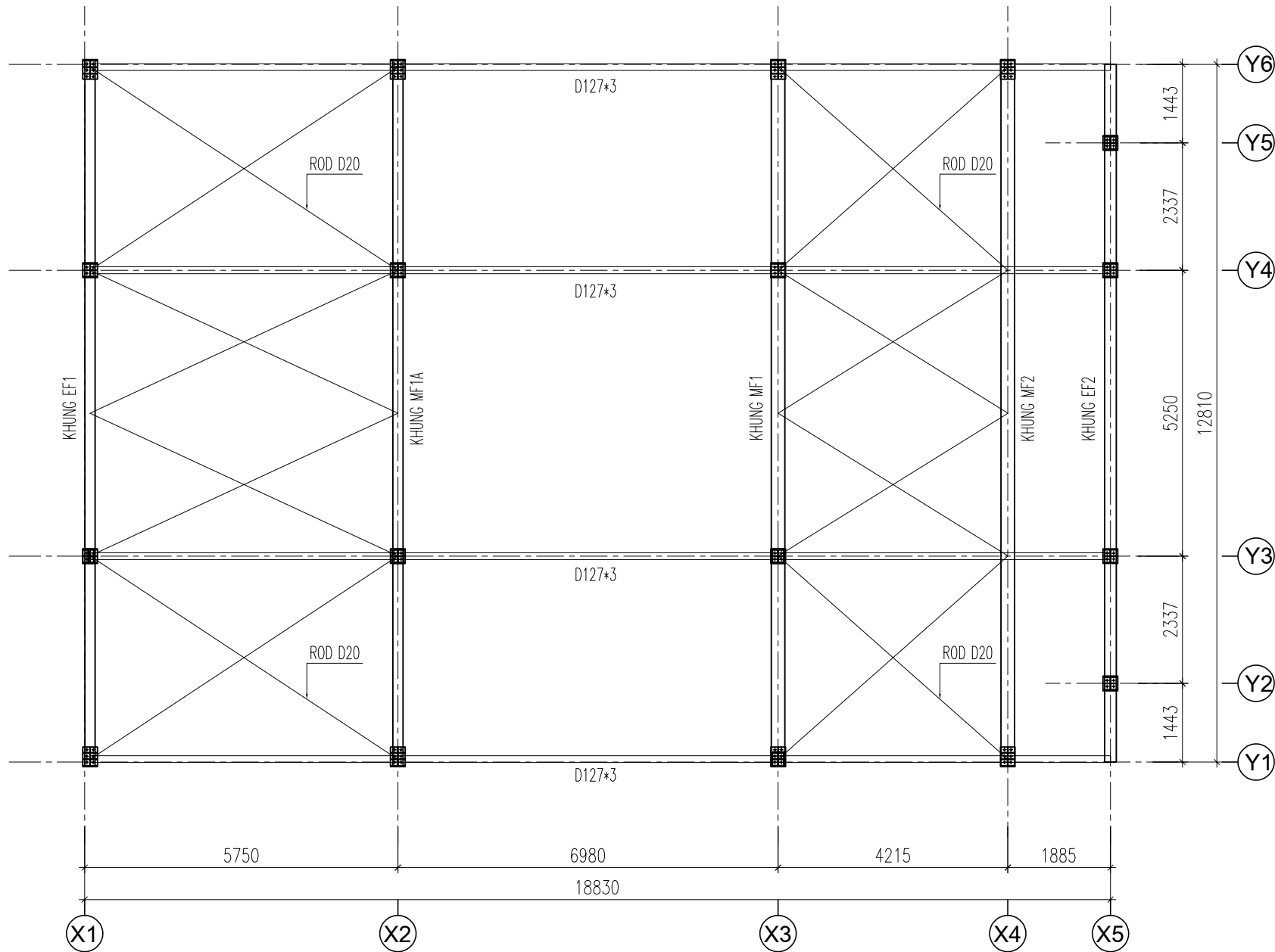
MẶT BẰNG KHUNG THÉP
