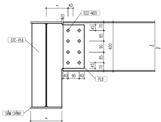
CHI TIẾT LIÊN KẾT DẦM PHỤ CHIỀU CAO H400*250
