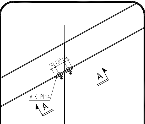
CHI TIẾT 7
