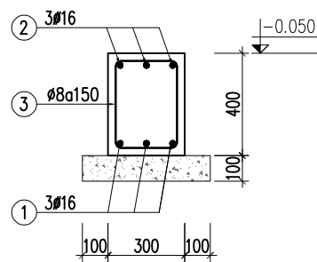
GM.6
