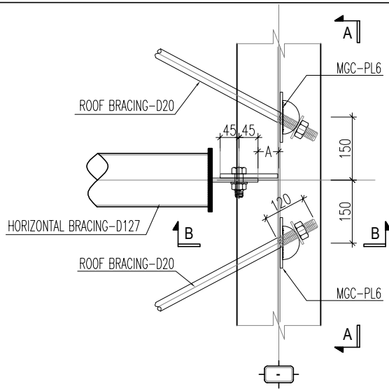
CHI TIẾT 1
