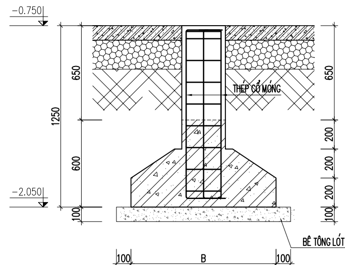
MẶT CẮT THÉP CỎ MÓNG
