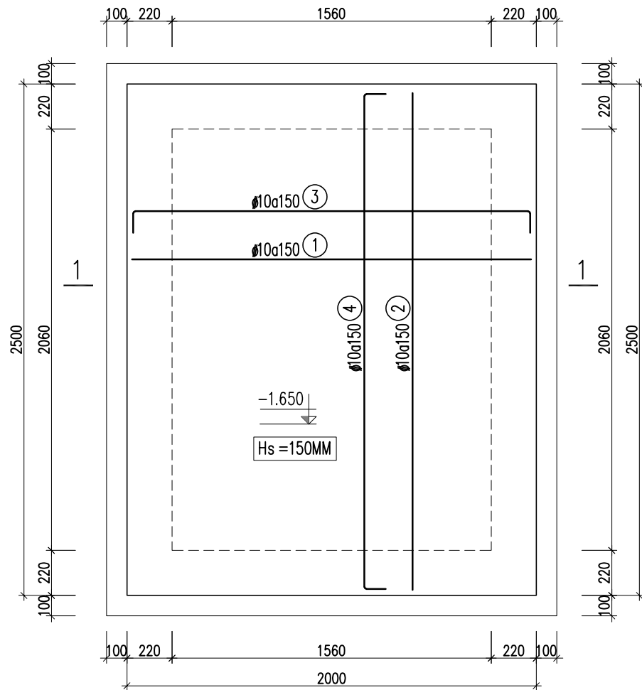
MẶT BẰNG BỐ TRÍ THÉP ĐÁY BỂ NƯỚC
