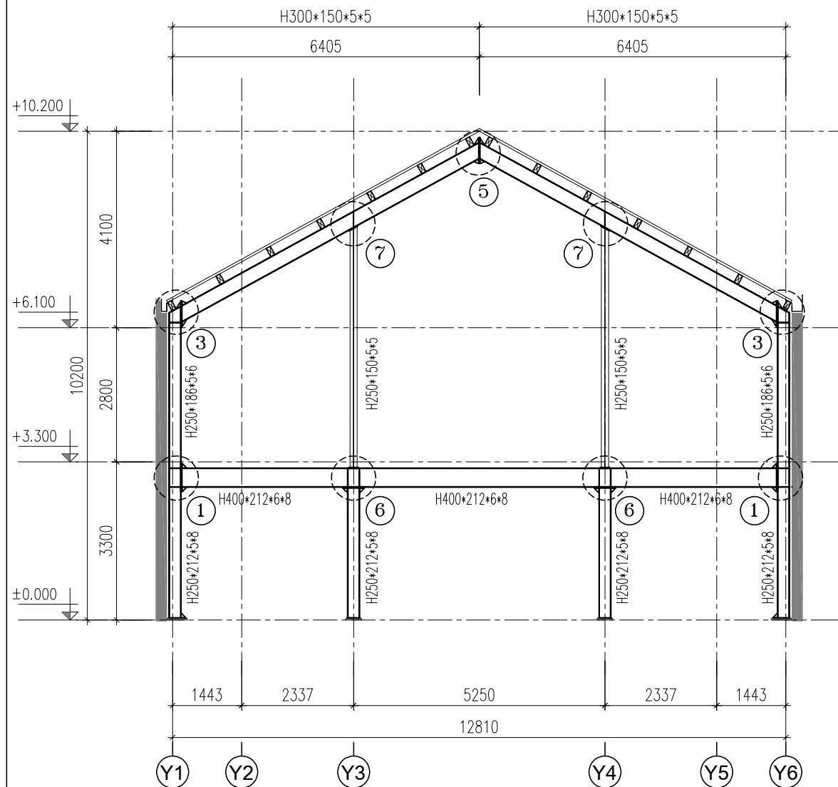
MẶT CẮT KHUNG EF1
