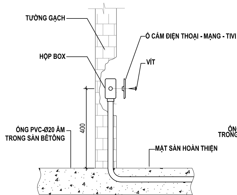
CHI TIẾT LẮP ĐẶT Ổ CĂM - CÔNG TẮC - ĐIỆN THOẠI - DATA - TIVI
