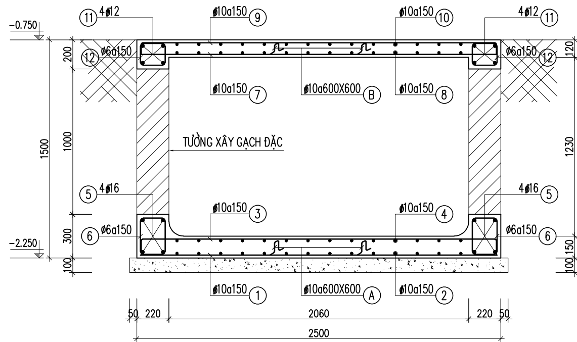
MẶT CẮT 1-1
