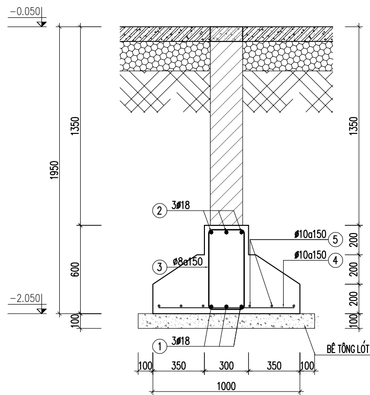
MÓNG MB.2
