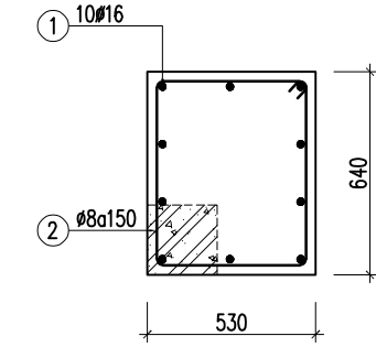
CM.4
