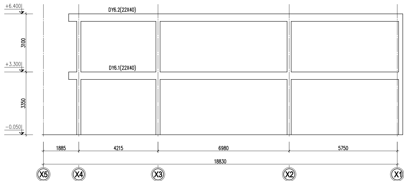
MẶT ĐỨNG KHUNG TRỤC Y6
