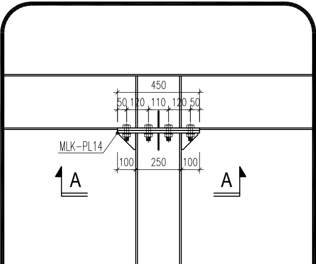
CHI TIẾT 9
