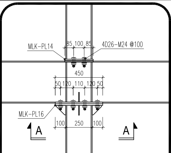
CHI TIẾT 2
