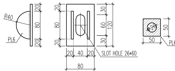
CHI TIẾT MÃ BÁN NGUYỆT
