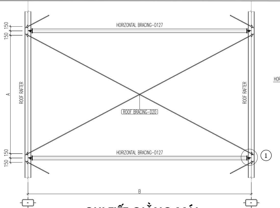
CHI TIẾT GIẪNG MÁI
