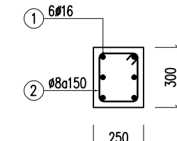
CM.5
