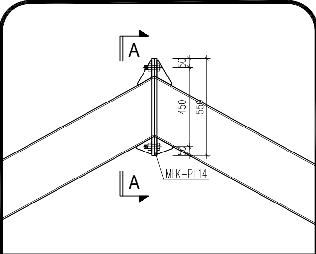
CHI TIẾT 11
