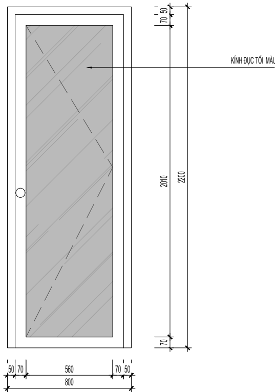
DW2 - 800X2200 - CỬA NHÔM KÍNH MỞ QUAY - SL 2
