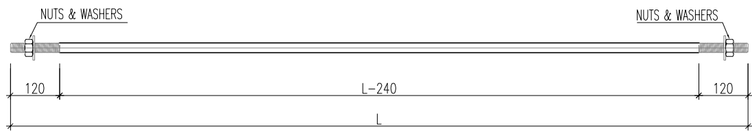
GIẪNG CHÉO D20
