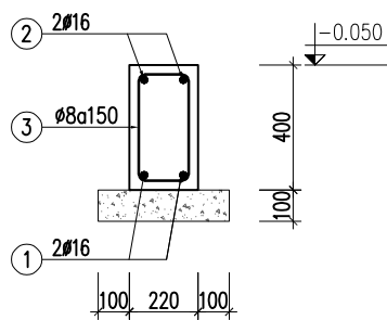
GM.5
