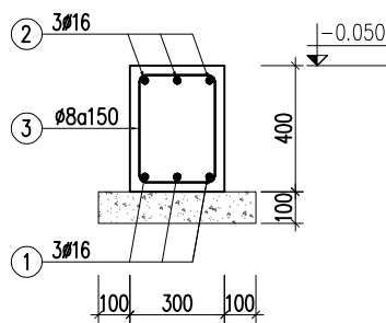
GM.4
