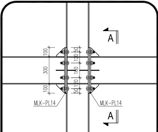
CHI TIẾT 8
