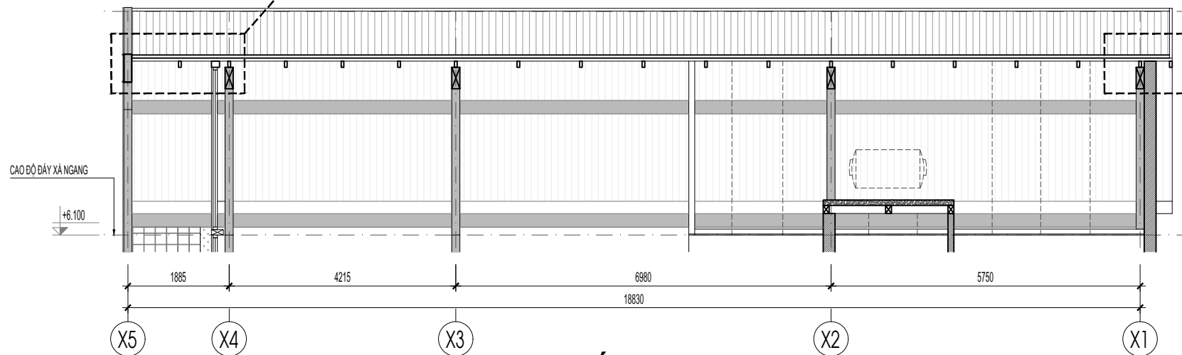
MẶT CẮT MÁI 2-2
