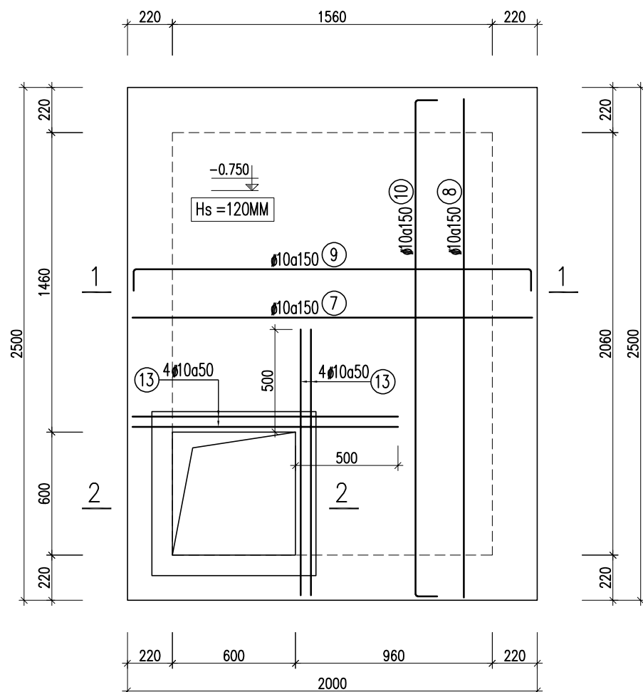
MẶT BẰNG BỐ TRÍ THÉP NẮP BỂ NƯỚC
