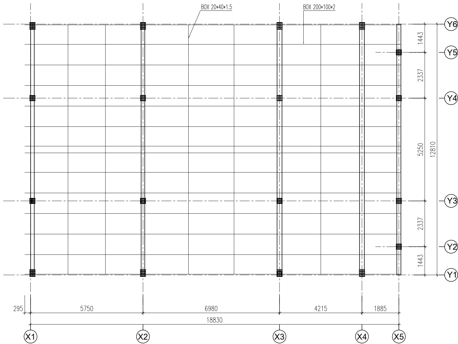
MẶT BẰNG XÀ GỖ MÁI
