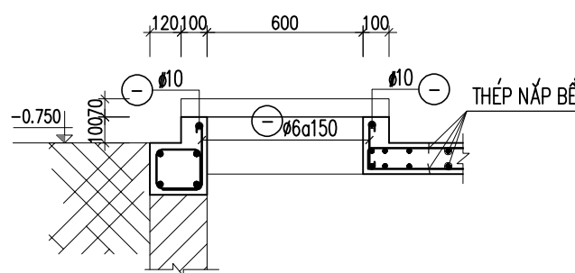
MẶT CẮT 2-2
