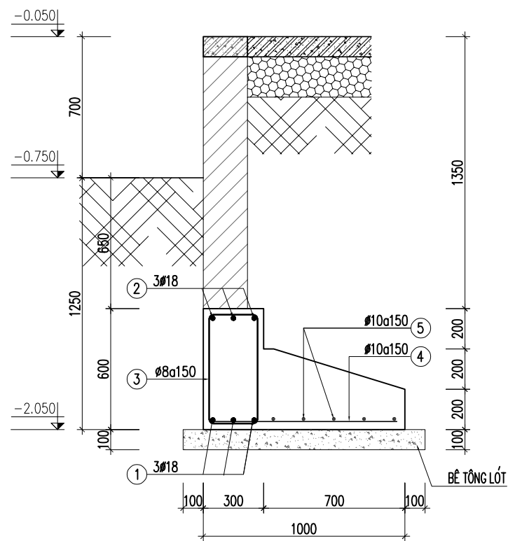
MÓNG MB.1
