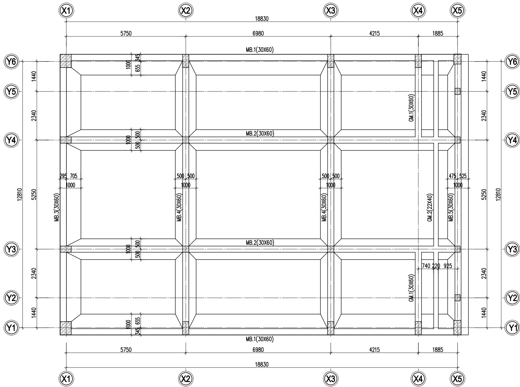
MẶT BẰNG BỐ TRÍ MÓNG
