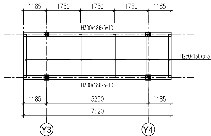
MẶT BẰNG SÀN KỸ THUẬT CỐT +6.650M
