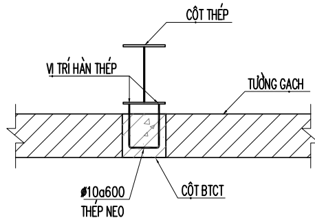
CHI TIẾT LÊN KẾT CỘT BTCT VÀ CỘT THÉP
