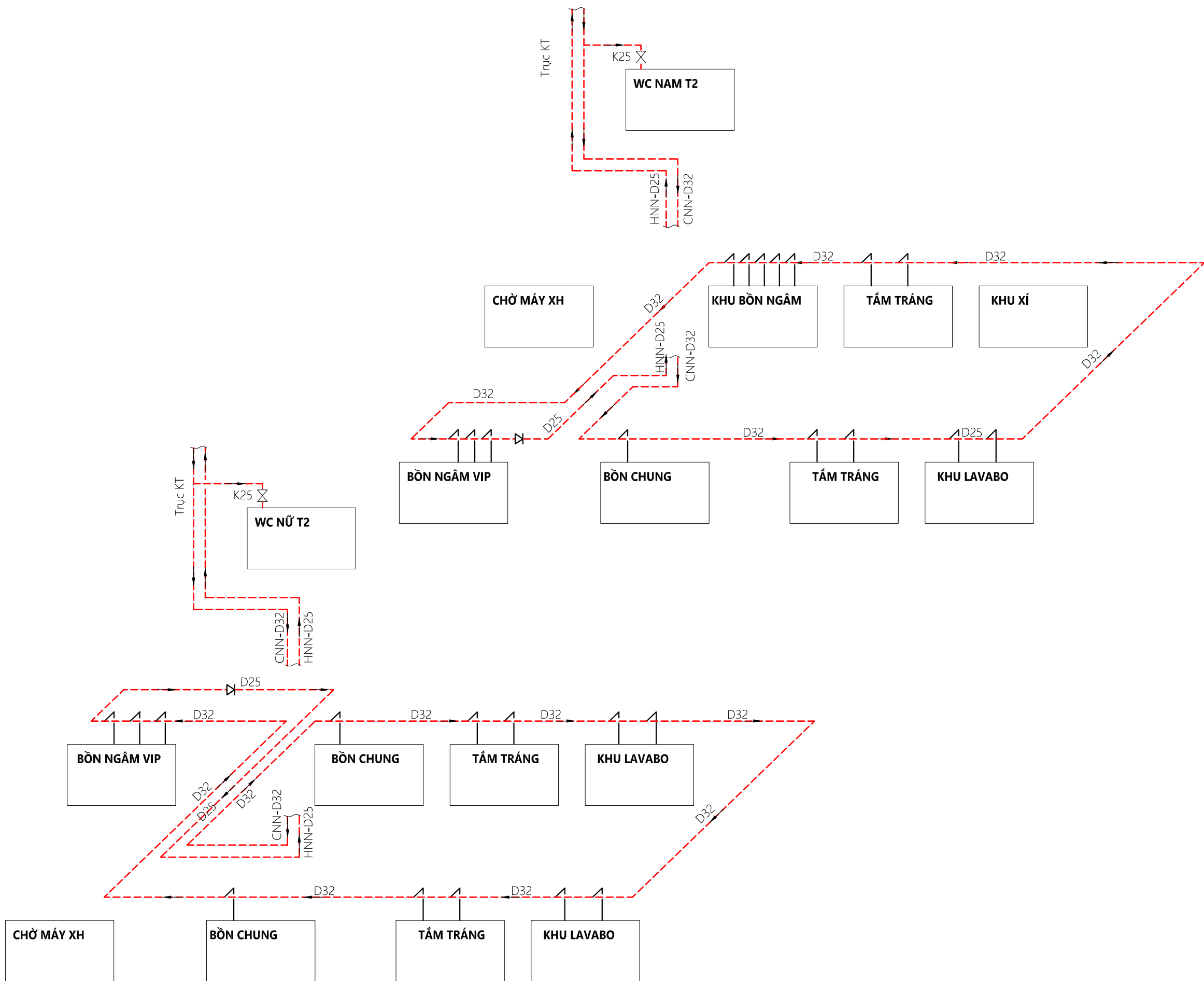
SƠ ĐỒ CẤP NƯỚC NÓNG
