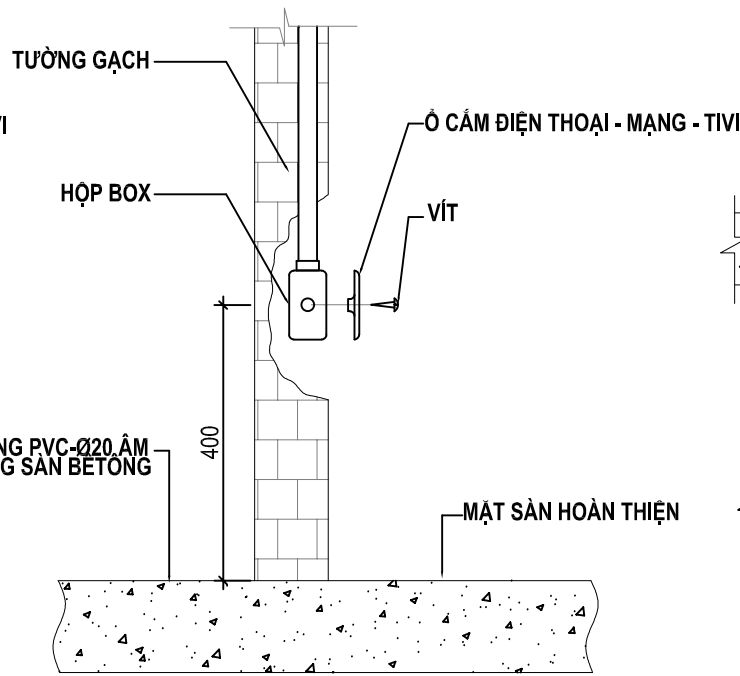
CHI TIẾT LẮP ĐẶT Ổ CĂM - CÔNG TẮC - ĐIỆN THOẠI - DATA - TIVI
