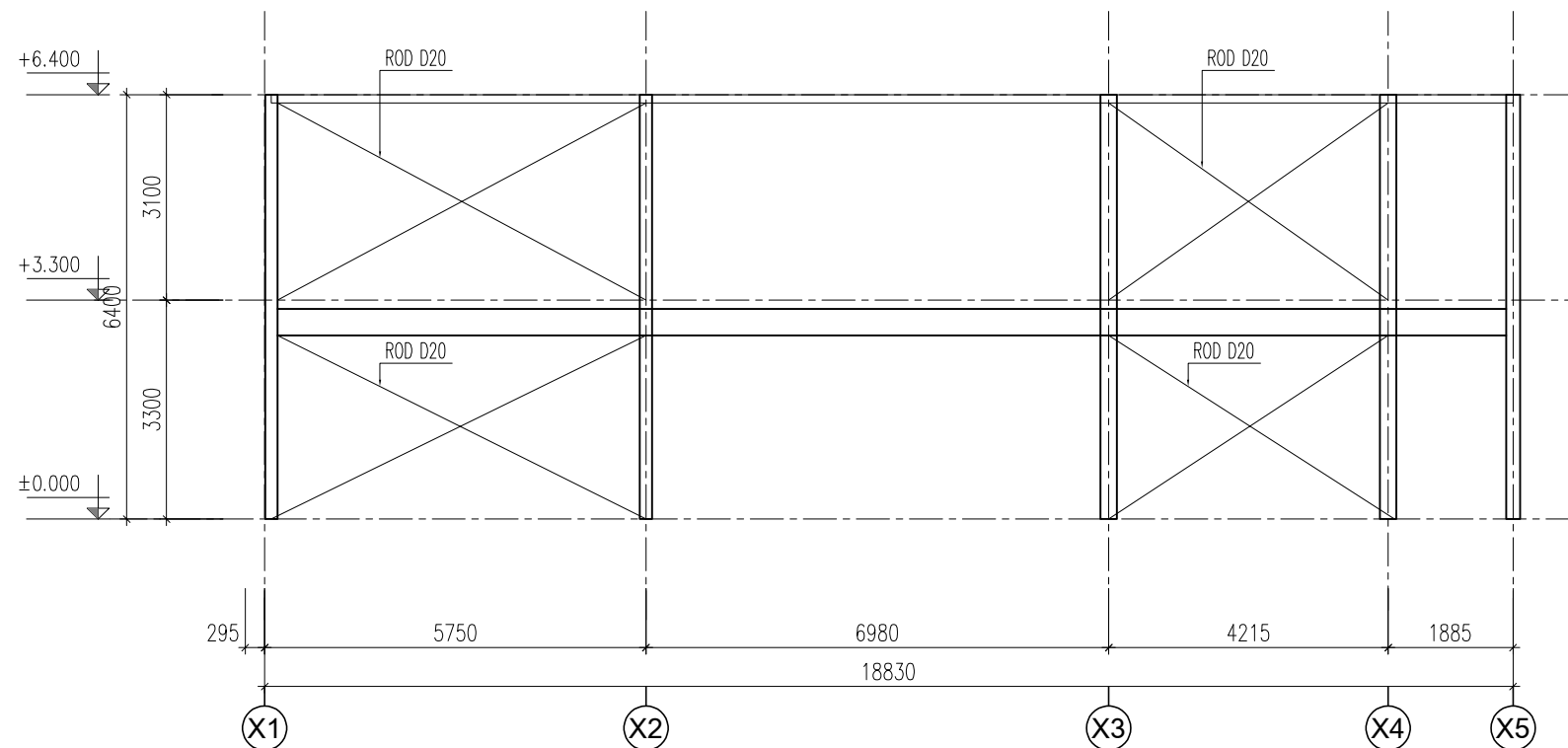
MẶT ĐÚNG GIẺNG CỘT TRỤC Y1 VÀ Y6
