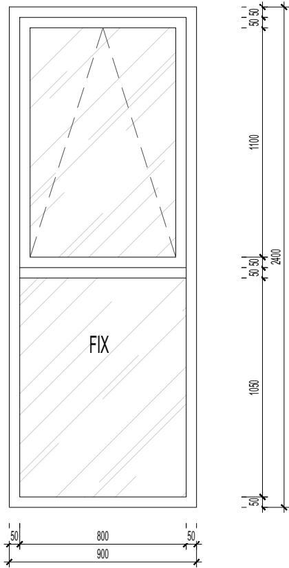
SVK2 - 900X2400 - VÁCH CỬA NHÔM KÍNH MỞ LẬT - SL 2
