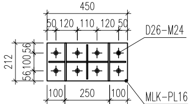
MẶT CẮT A-A
