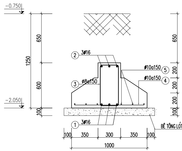
MÓNG MB.5
