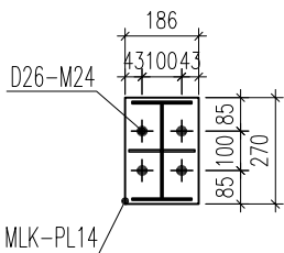
CHI TIẾT 7
