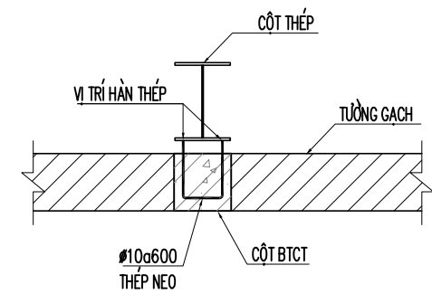
CHI TIẾT LÊN KẾT CỘT BTCT VÀ CỘT THÉP
