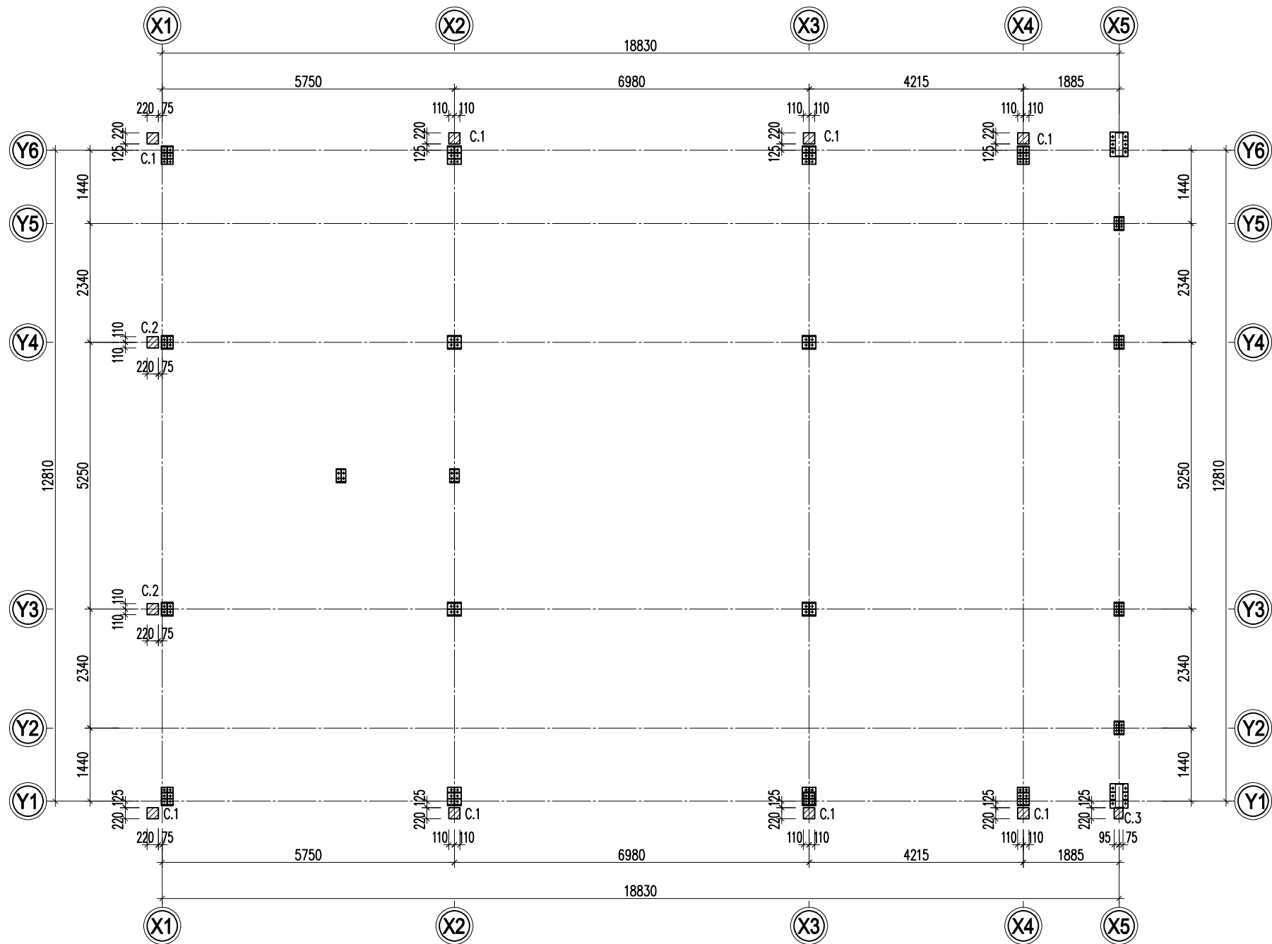
MẶT BẰNG ĐỊNH VỊ CỘT
