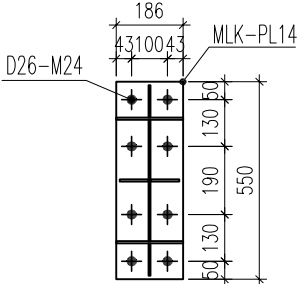
MẶT CẮT A-A
