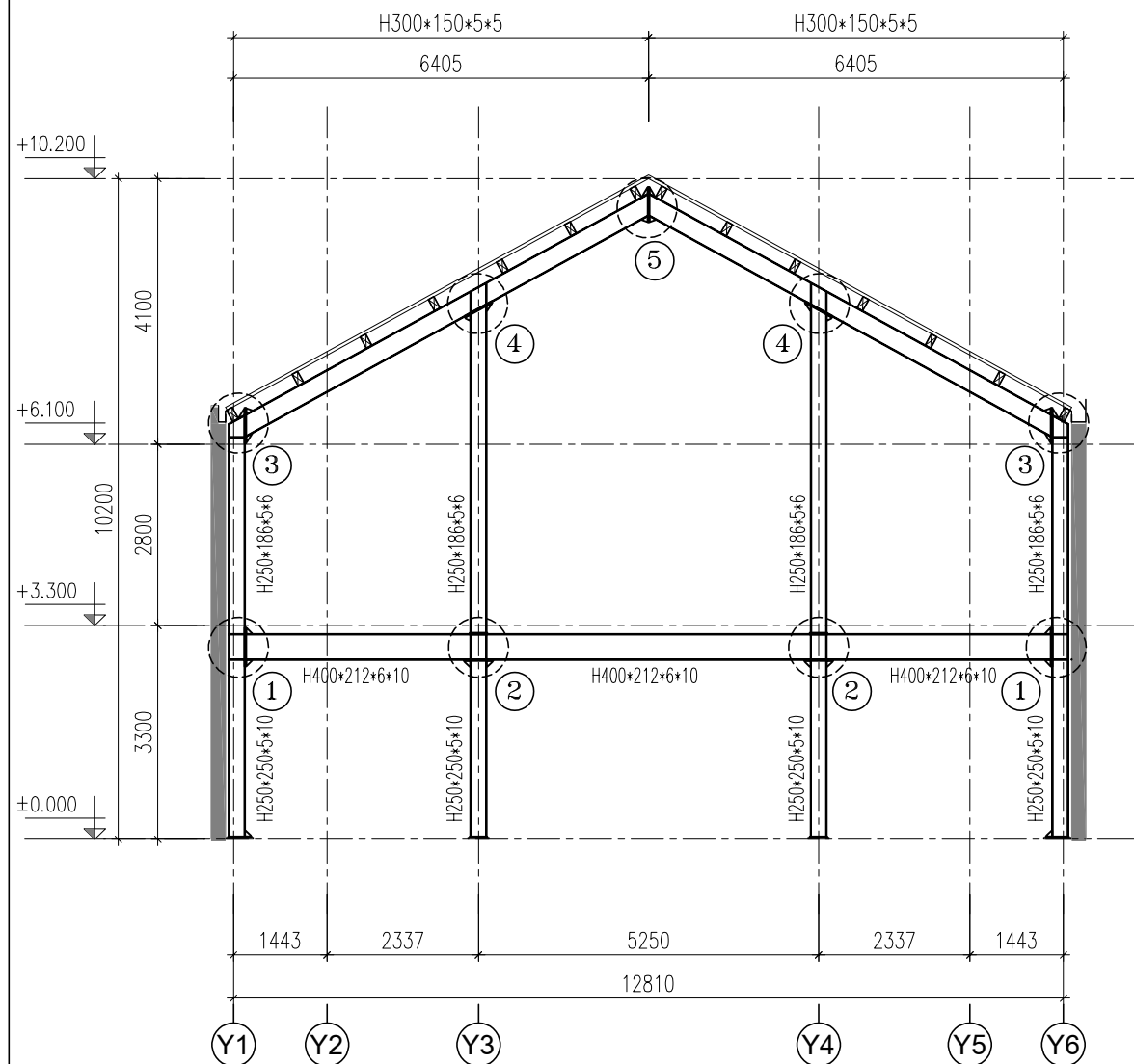
MẶT CẮT KHUNG MF1
