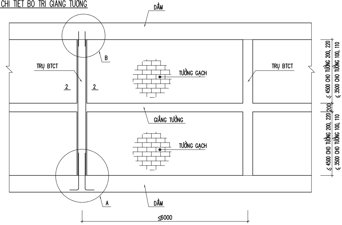
GIẺNG TƯỜNG 110
