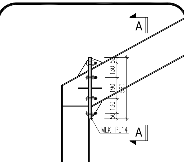
CHI TIẾT 3
