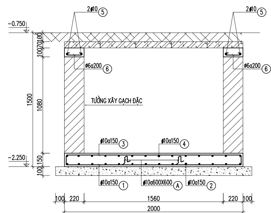
MẶT CẮT 1-1
