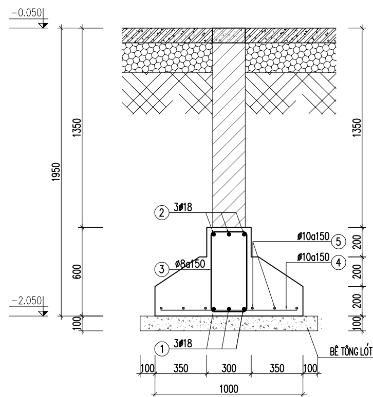
MÓNG MB.4
