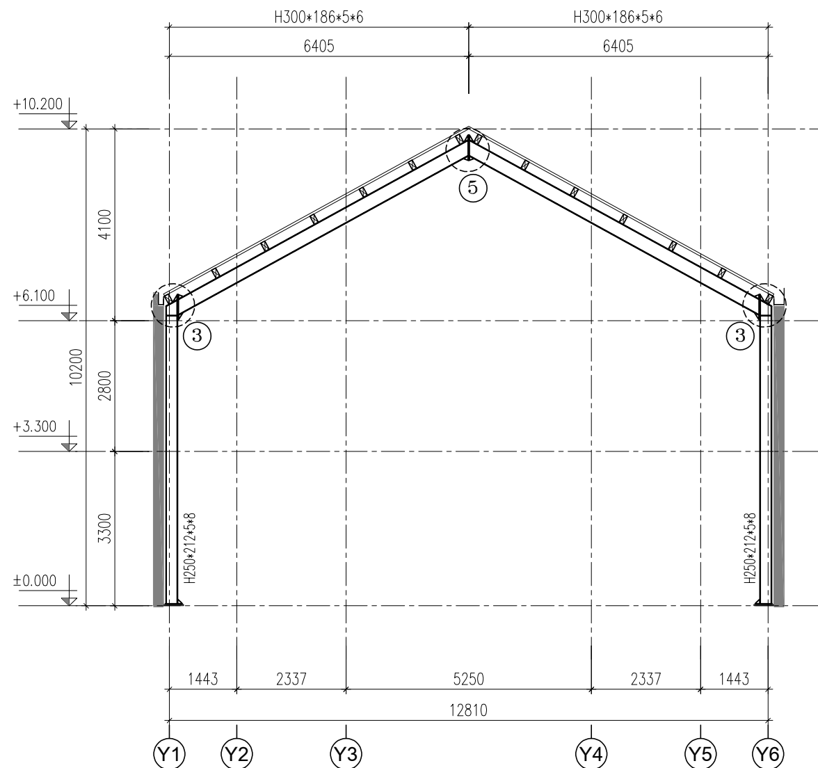
MẶT CẮT KHUNG MF2
