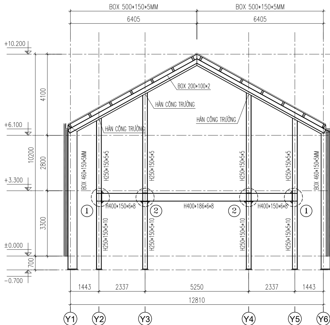
MẶT CẮT KHUNG EF2
