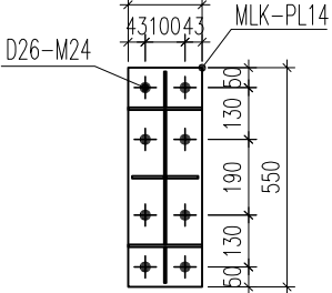
MẶT CẮT A-A
