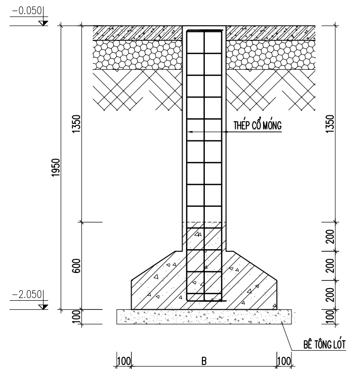
MẶT CẮT THÉP CỎ MÓNG
