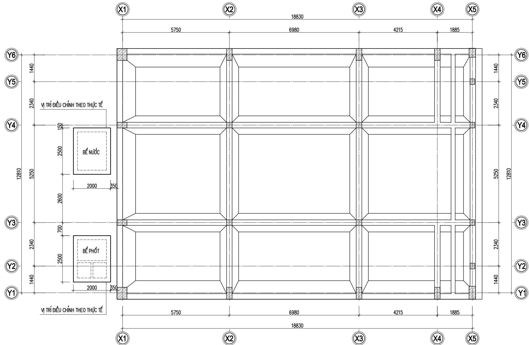
MẶT BẰNG BỐ TRÍ BỂ NƯỚC, BỂ PHỐT
