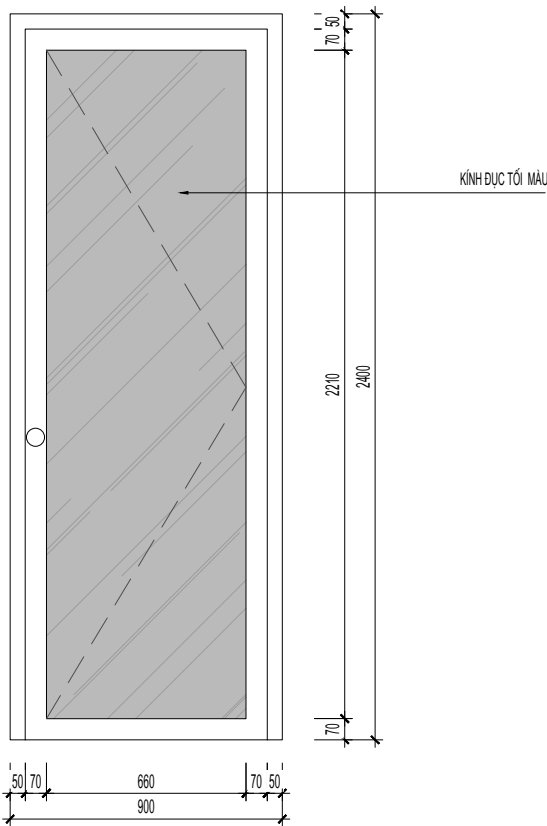
D2 - 900X2400 - CỬA NHÔM KÍNH MỞ QUAY - SL 4
