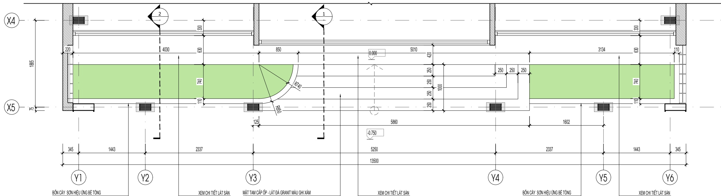
MẶT BẰNG TAM CẤP - BỒN CÂY
