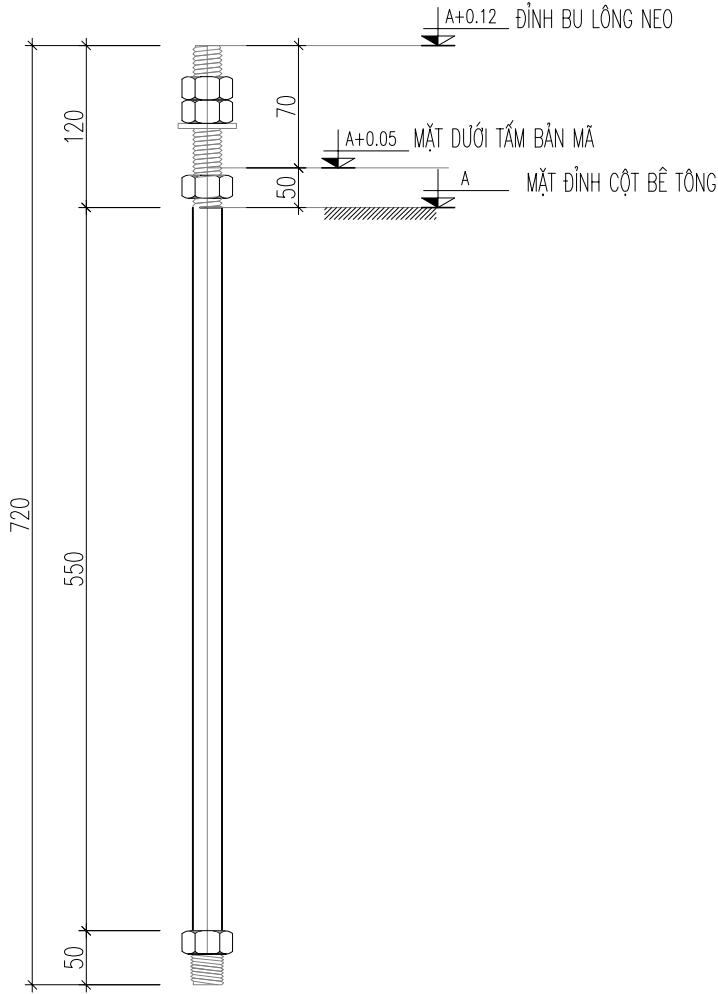
BU LÔNG NEO : M20*720 GRADE: 5.6
