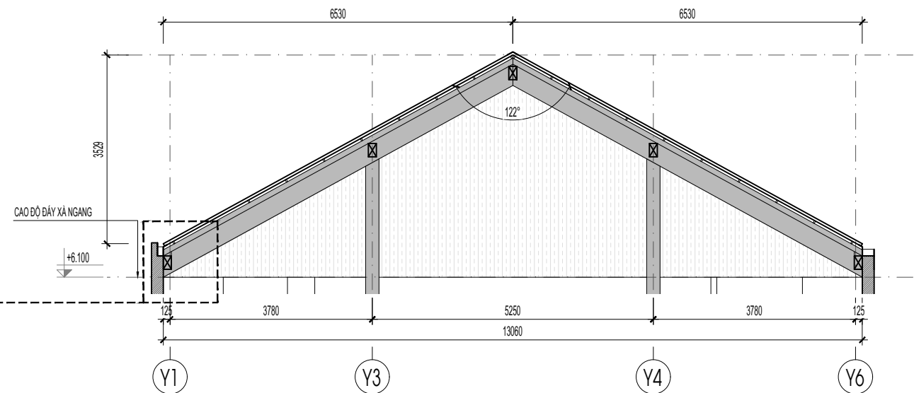
MẶT CẮT MÁI 1-1
