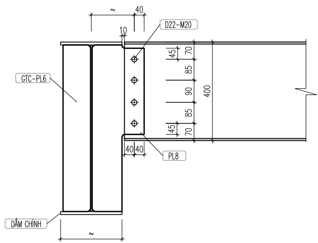
CHI TIẾT LIÊN KẾT DẦM PHỤ CHIỀU CAO H400*186
