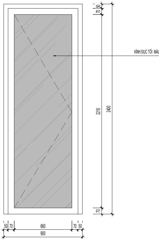
DW1 - 900X2400 - CỬA NHÔM KÍNH MỞ QUAY - SL 4
