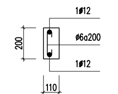
GIẺNG TƯỜNG 110
