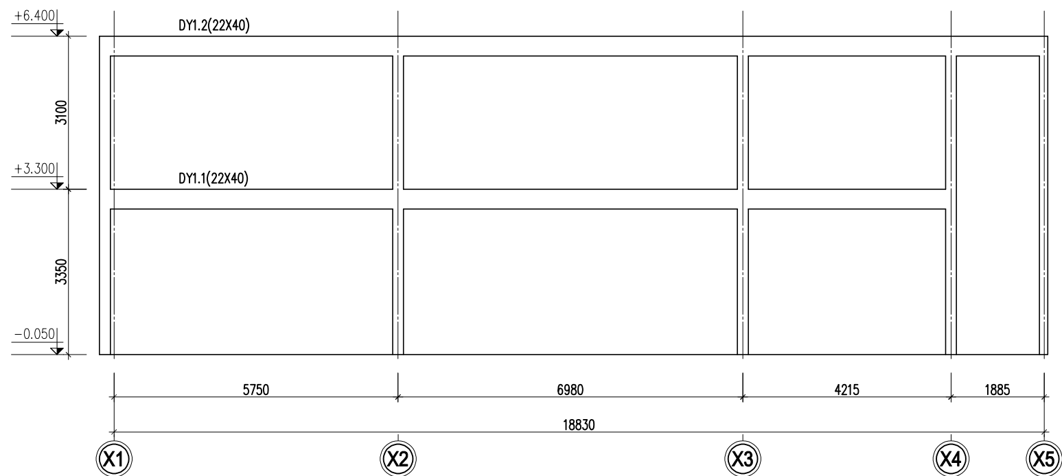
MẶT ĐỨNG KHUNG TRỤC Y1
