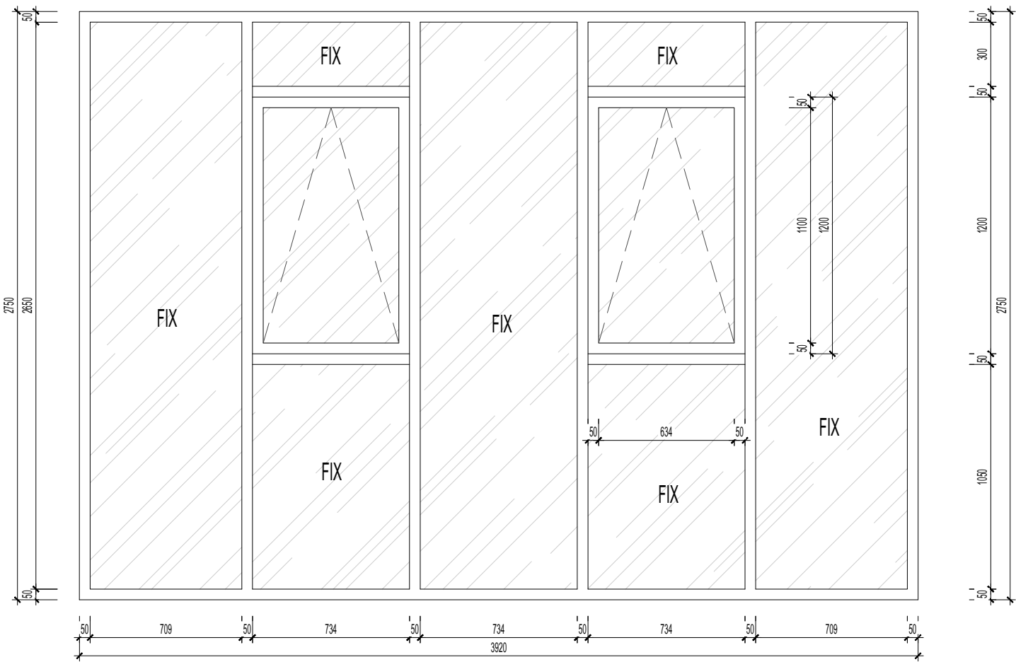
SVK1 - 3920X2750 - VÁCH CỬA NHÔM KÍNH MỞ LẬT - SL 2
